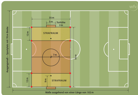
Kleinspielfeld für zwei tragbare Tore 5 x 2 m
